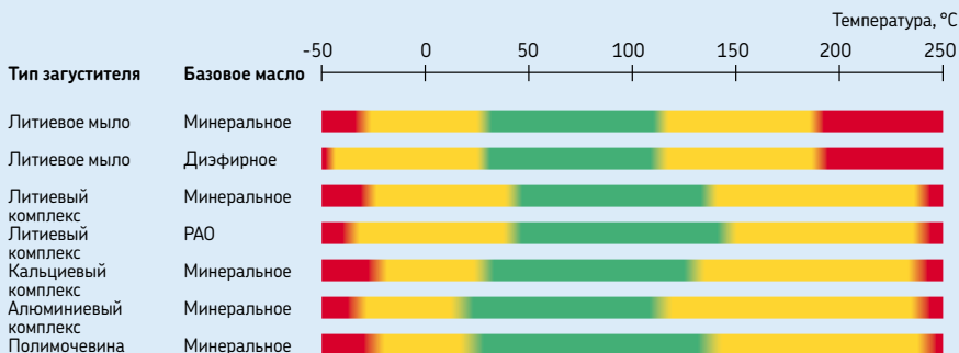
Принцип светофора SKF – стандартные пластичные смазки
